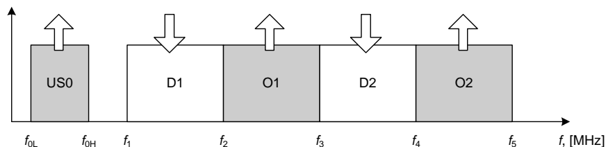
Slika 4.8.1 Frekventijski plan za pojas prijenosa do 12 MHz (G.993.2)
